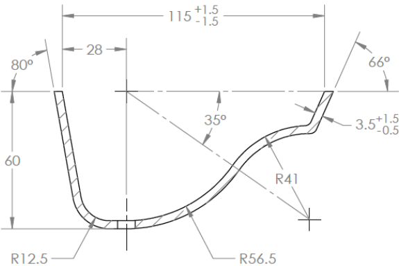
SECTION B-B SCALE 2 : 3
