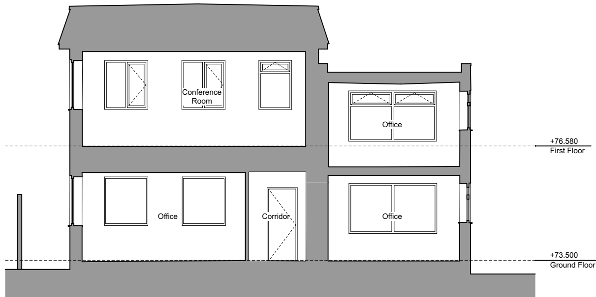
2 Section DD 1:100
