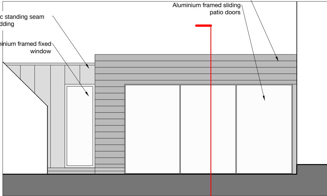
Elevation - 1:50
