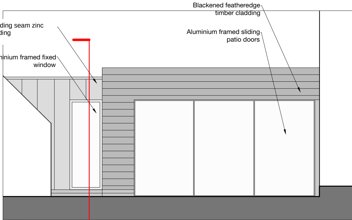
Elevation - 1:50
