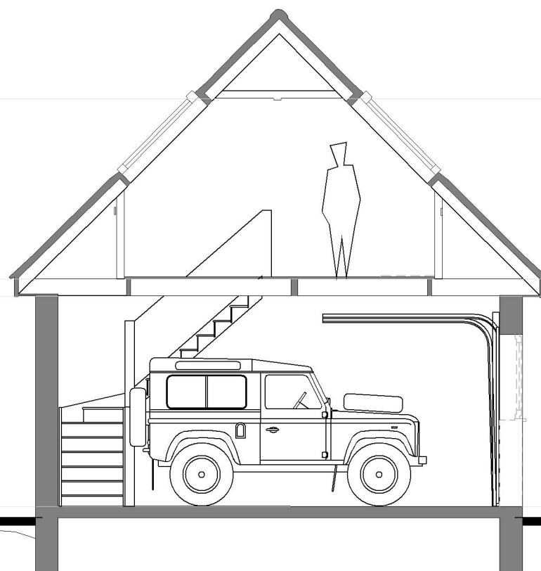
SECTION A-A
