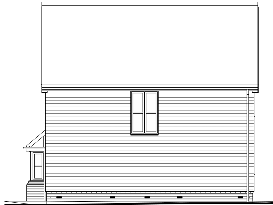
Right Elevation
