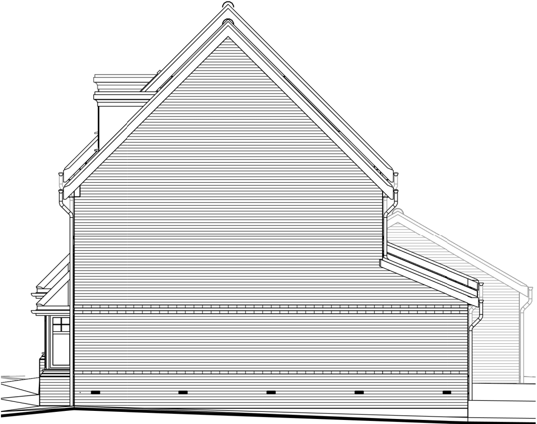
Right Elevation
