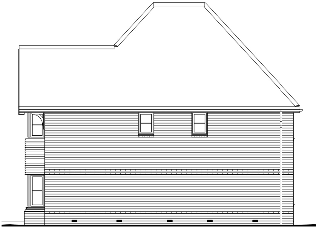
Right Elevation
