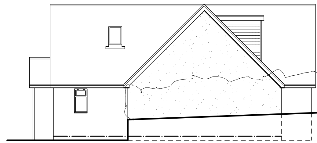
SW ELEVATION
