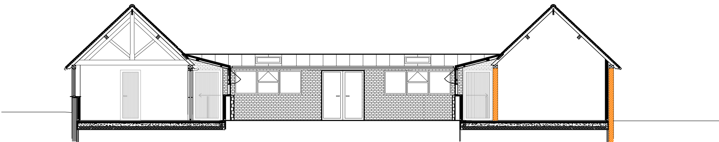
SECTION D-D
