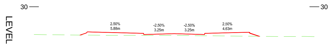
NORTHERN ARC AVENUE CL-1140.000 SCALE: H 1:200,V 1:200. DATUM: 22.500
