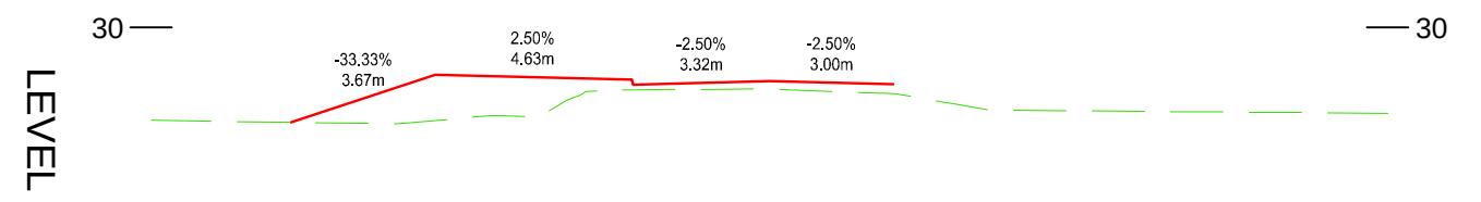
ROAD 08-102.575 SCALE: H 1:200,V 1:200. DATUM: 22.500
