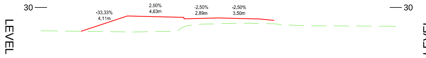
ROAD 08-80.000 SCALE: H 1:200,V 1:200. DATUM: 22.500
