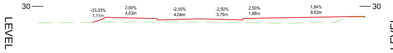
ROAD 08-33.534 SCALE: H 1:200,V 1:200. DATUM: 22.500
