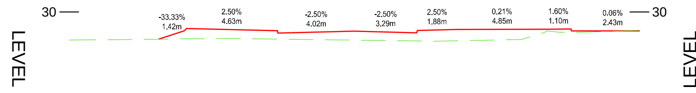
ROAD 08-40.000 SCALE: H 1:200,V 1:200. DATUM: 22.500
