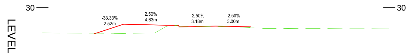
ROAD 08-120.000 SCALE: H 1:200,V 1:200. DATUM: 22.500
