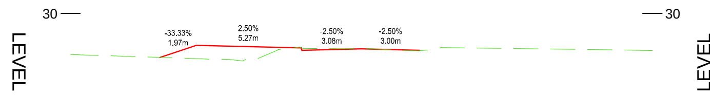
ROAD 08-140.000 SCALE: H 1:200,V 1:200. DATUM: 22.500
