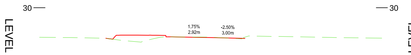
ROAD 08-192.216 SCALE: H 1:200,V 1:200. DATUM: 22.500
