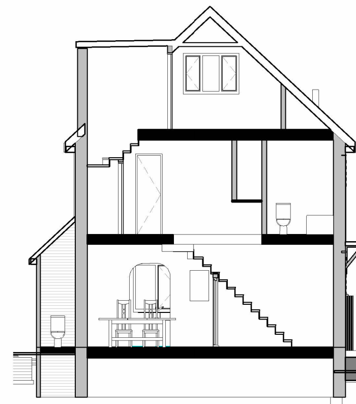
5 Section 2 1 : 100
