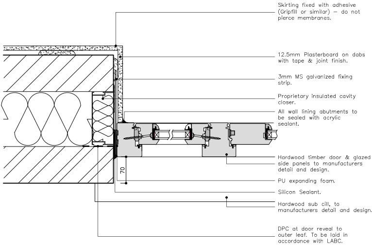
TIMBER DOOR JAMB DETAIL
