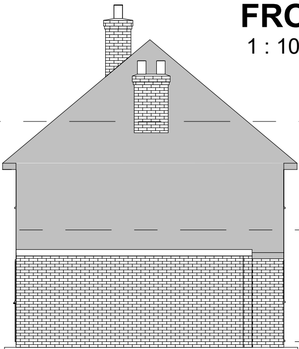
ELEVATION 'B'
