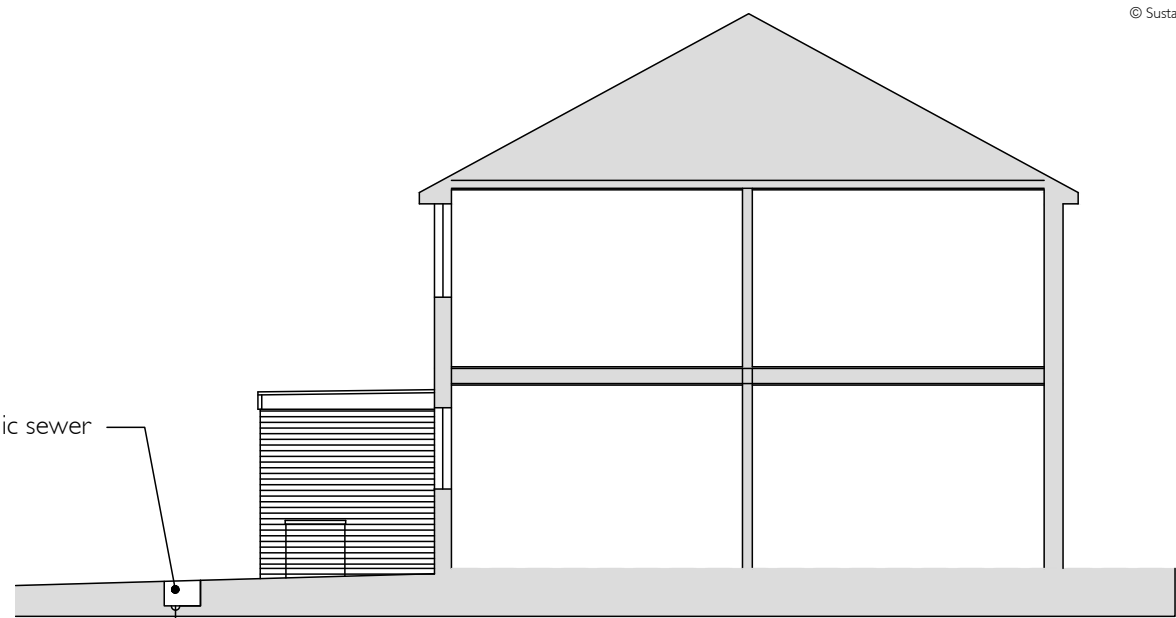
existing section a-a 1:100
