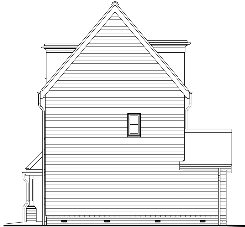
Right Elevation
