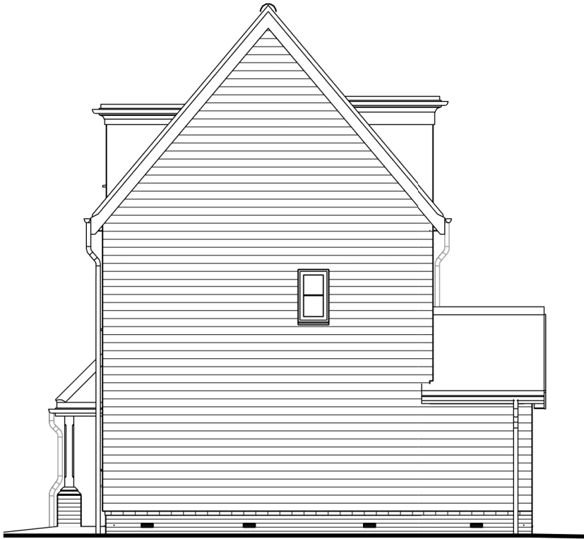
Right Elevation
