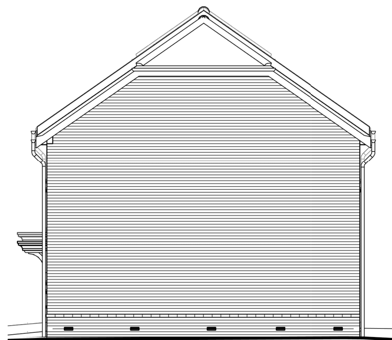
Right Elevation
