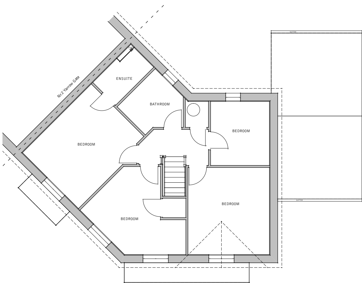
2 1F Plan Scale: 1:100
