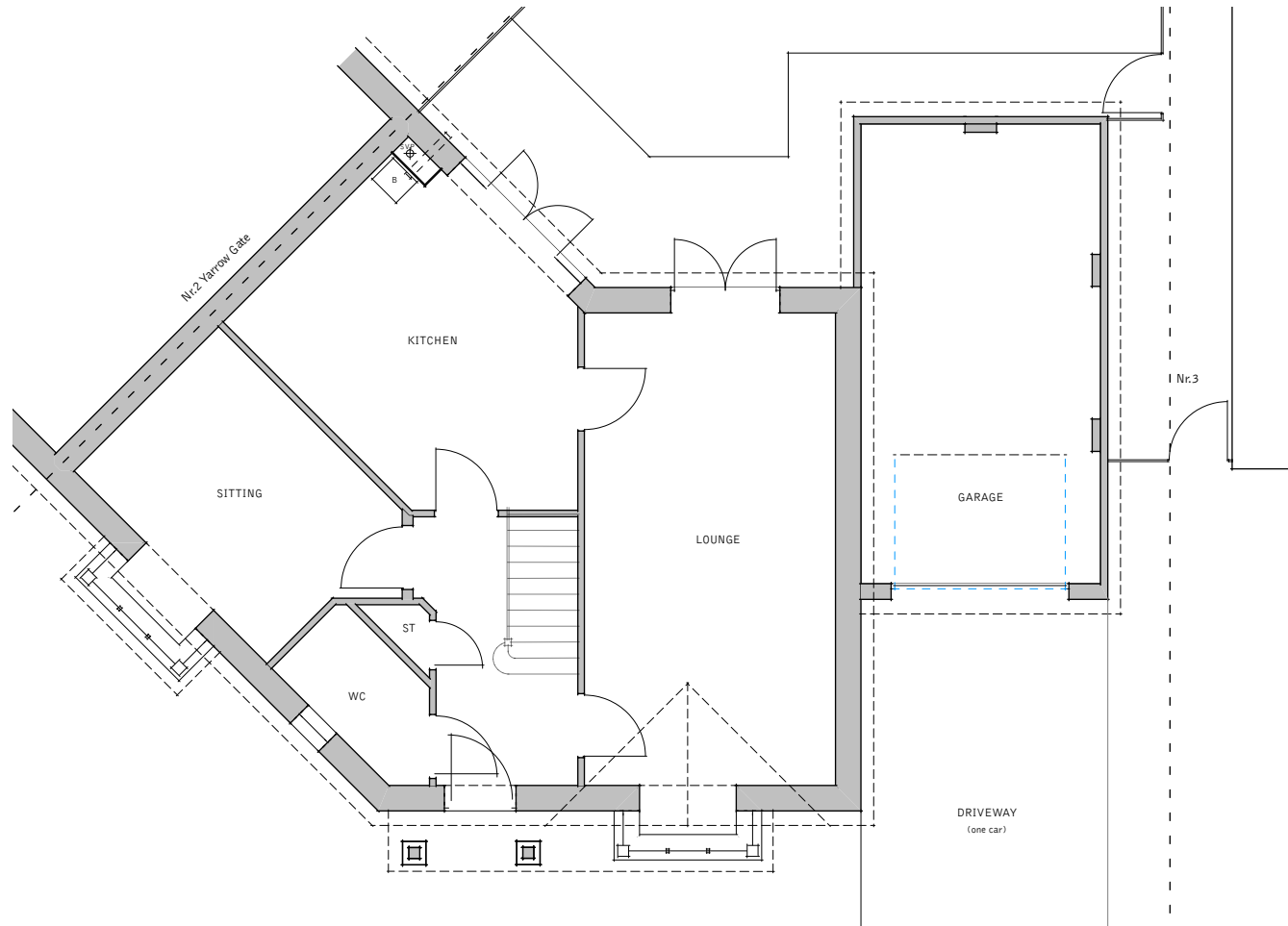
1 GF Plan Scale: 1:100
