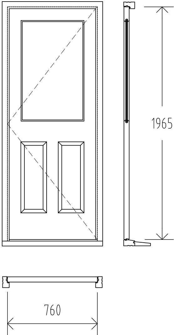
Side Entrance Door door 760 (w) x 1965 (h) frame 850 (w) x 2065 (h)
