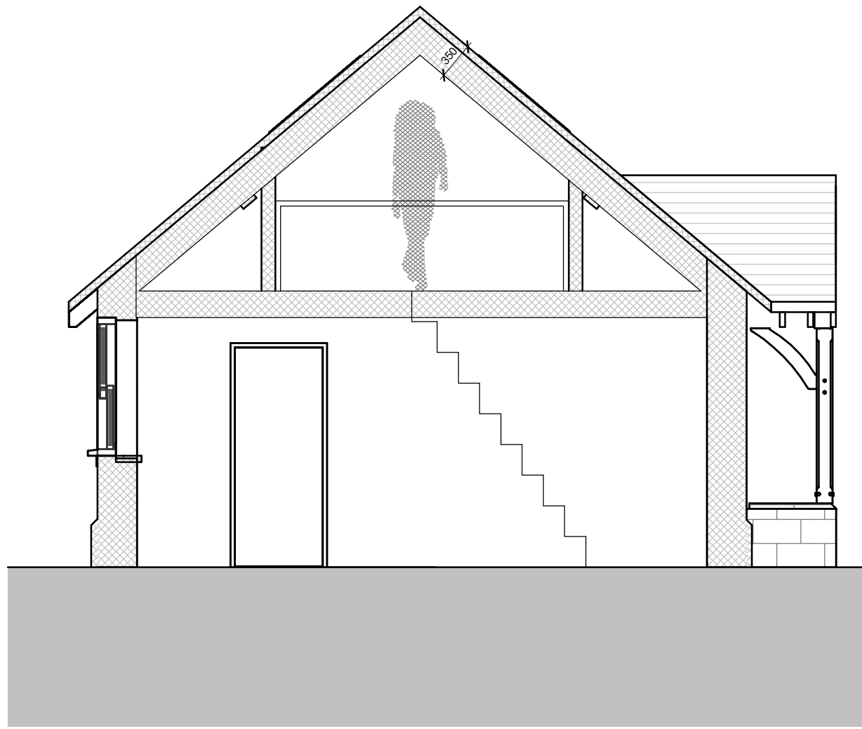
Section A-A 1 : 50
