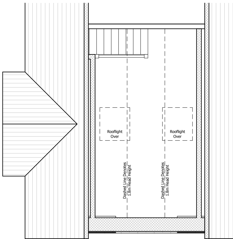
Mezzanine 1 : 50
