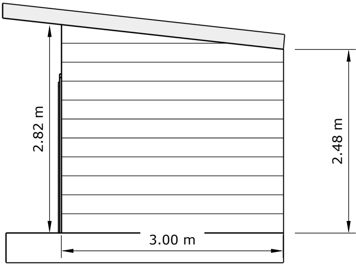
SIDE ELEVATION SE
