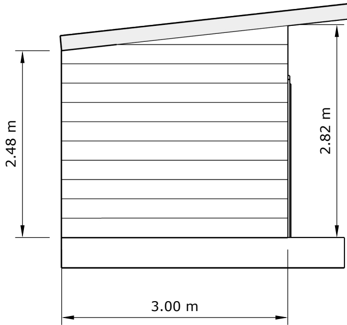
SIDE ELEVATION SE
